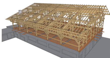
3D-PLAN
